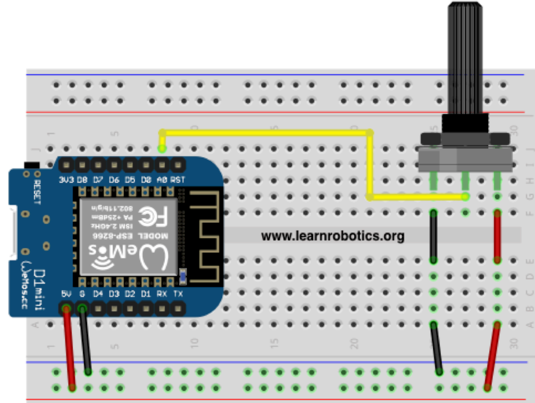
مخطط التوصيل الفيزيائي
